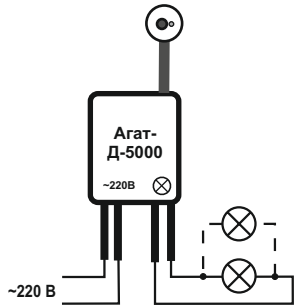
Рис.1. Схема монтажа
