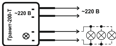
Рис.1. Схема монтажа для ламп 220 В
